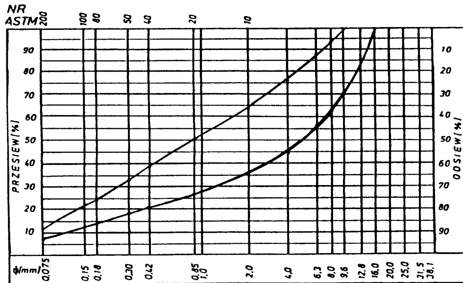
Rys. 3. Krzywe graniczne uziarnienia mieszanki mineralnej 0+8, 0+6,3 mm do warstwy ścieralnej z betonu asfaltowego dla KR 2
