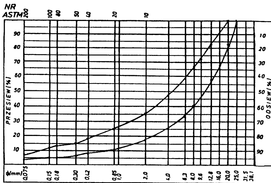
Rys. 1. Krzywe graniczne uziarnienia mieszanki mineralnej 0+31,5 mm do podbudowy z betonu
