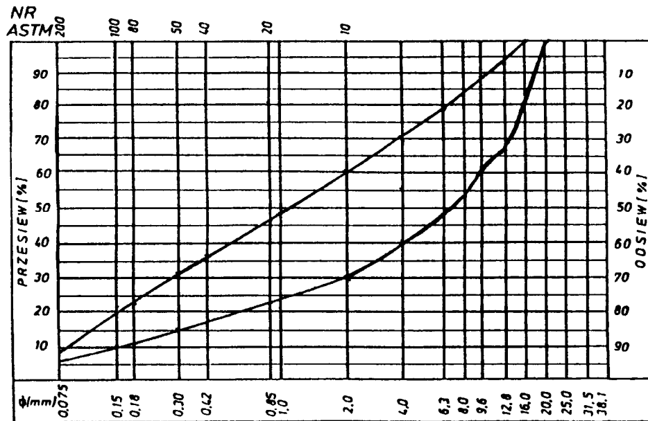
Rys. 1. Krzywe graniczne uziarnienia mieszanki mineralnej 0+20 mm do warstwy ścieralnej z betonu asfaltowego dla KR 2
