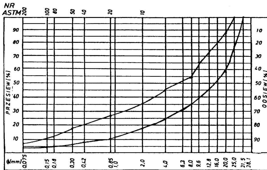
Rys. 1. Krzywe graniczne uziarnienia mieszanki mineralnej 0+31,5 mm do podbudowy z betonu
