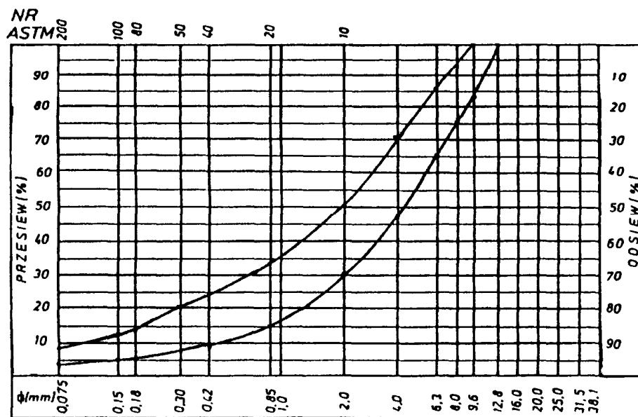
Rys. 5. Krzywe graniczne uziarnienia mieszanki mineralnej 0÷12,8 mm do podbudowy z betonu
