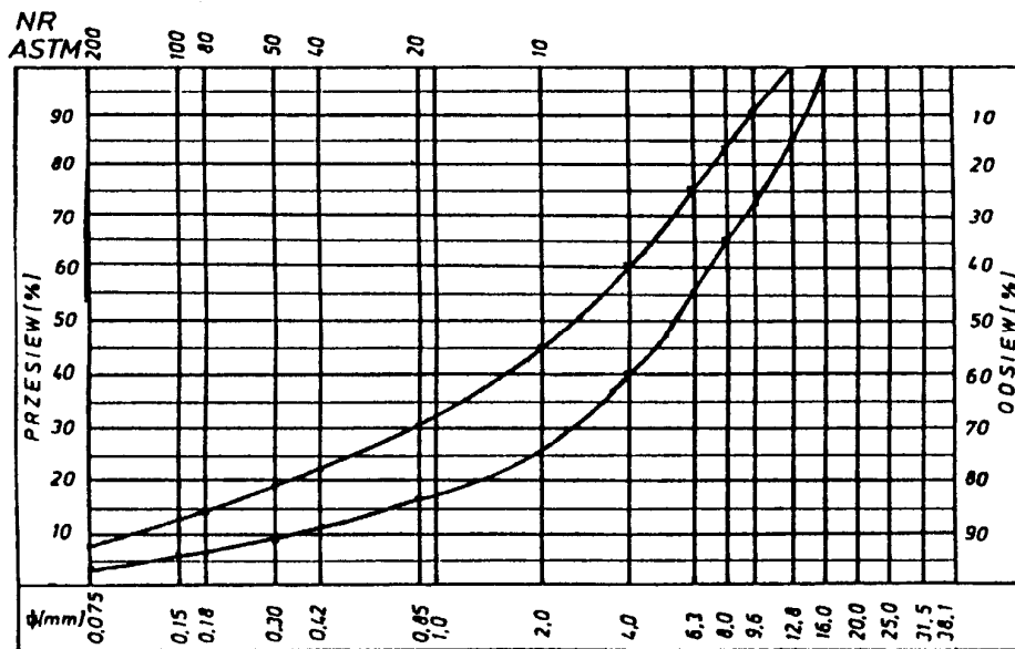
Rys. 3. Krzywe graniczne uziarnienia mieszanki mineralnej 0÷20 mm do podbudowy z betonu
