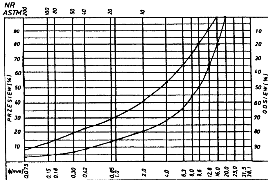
Rys. 3. Krzywe graniczne uziarnienia mieszanki mineralnej 0÷20 mm do podbudowy z betonu
